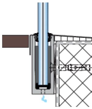
Stirnseitige Montage
