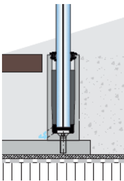
Aufgesetzte Montage
